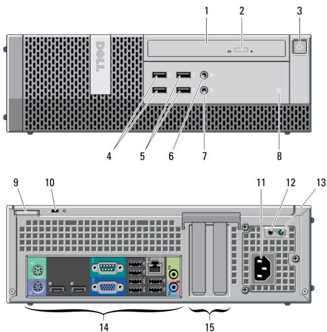
Obrázok 3. Pohľad na predný a zadný panel modelu Small Form Factor
